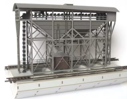
Art.-Nr. Z10301: Hunt'sche Großbekohlungsanlage Bauart Antwerpen
